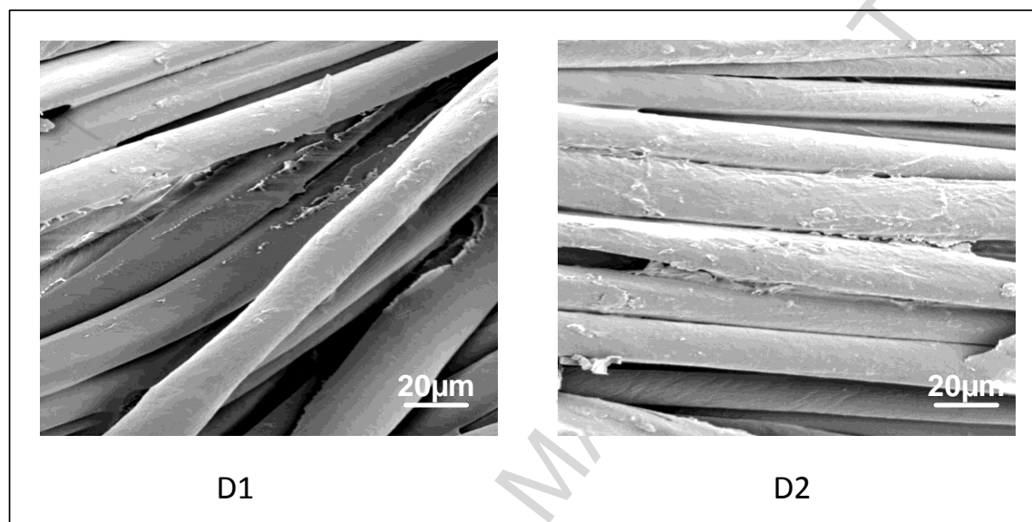
Figure 6: SEM of D1 and D2
