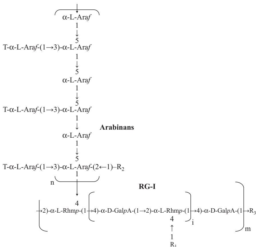
Fig. 4.8 Rhamnogalacturonan I (RGI)
