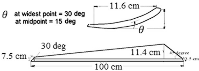
Fig. 29.6 Blade dimensions
